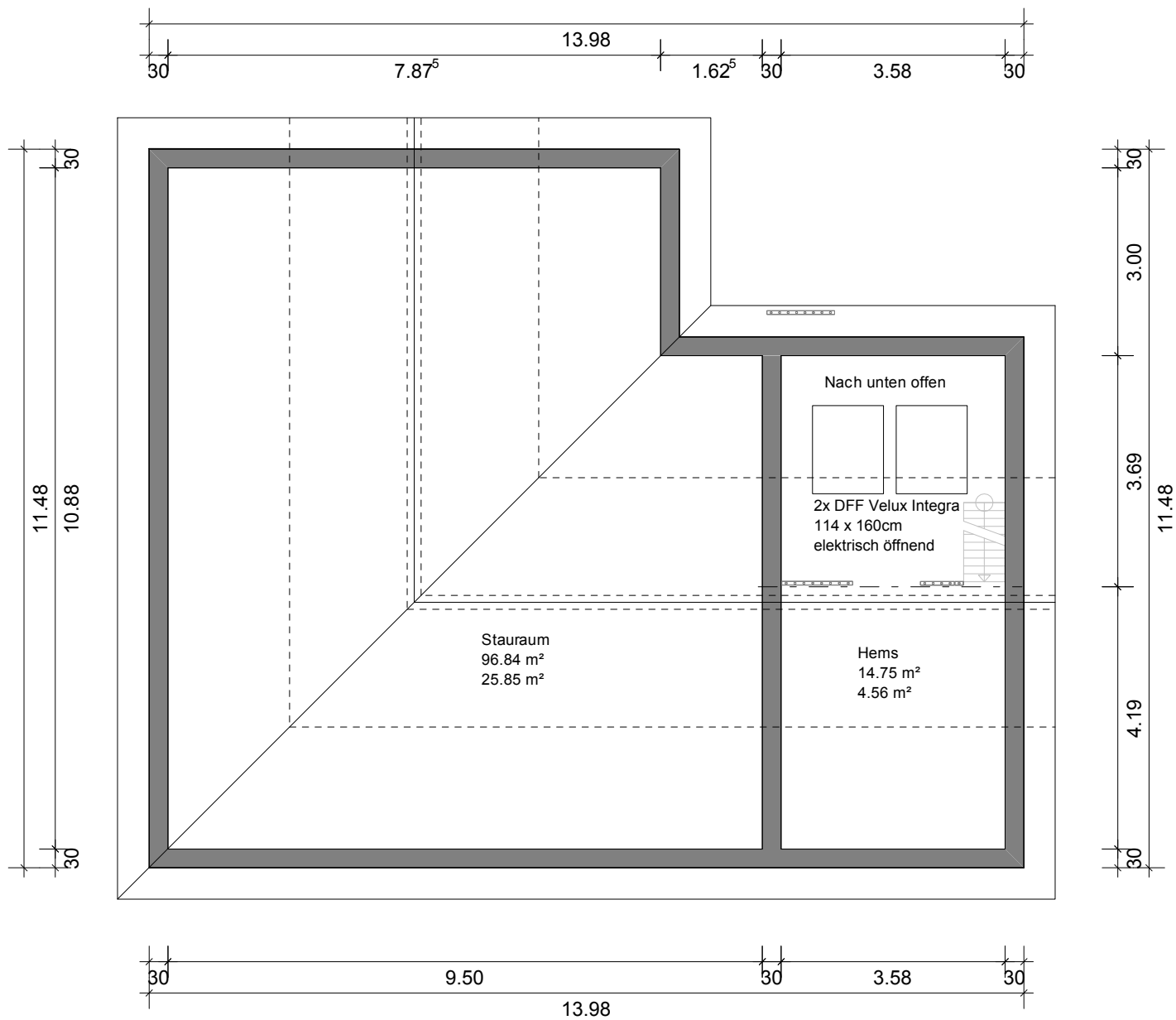
Bungalowplanung mit Hems und offenem Bereich über dem Esszimmer
